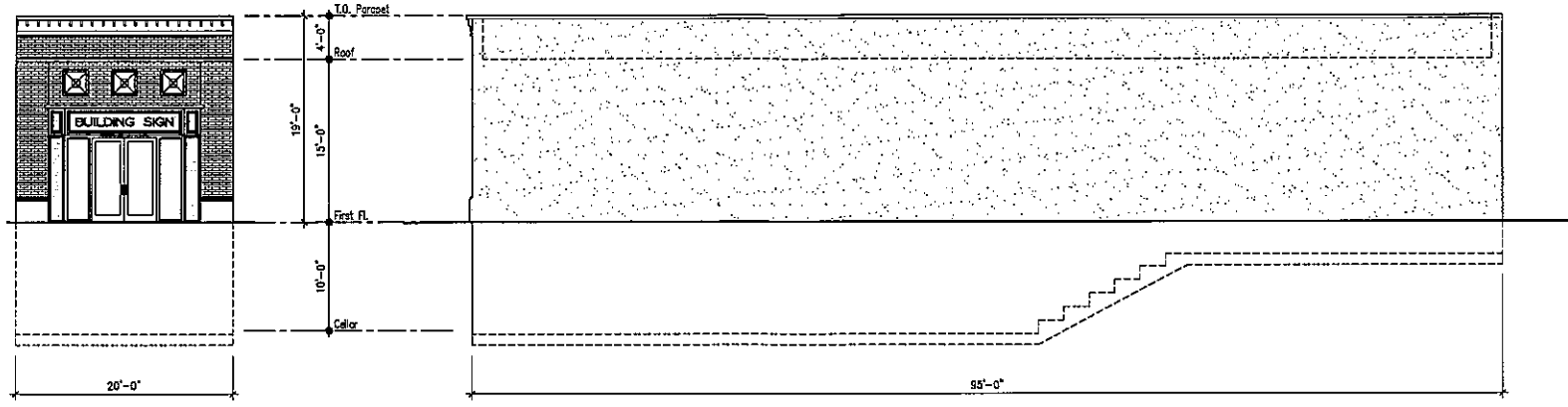
FRONT ELEVATION SCALE: 1/8" = 1'-0"
