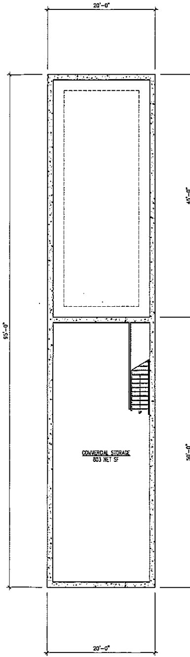
CELLAR PLAN SCALE: 1/8" = 1'-0"
